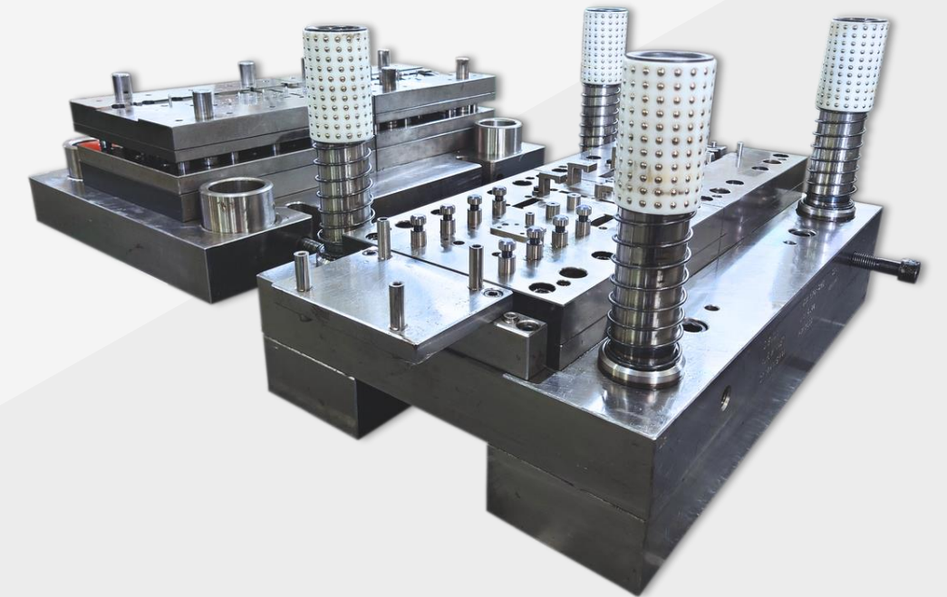
Progressive Die
